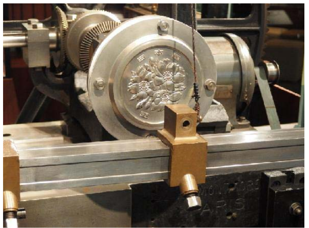
錢幣雕刻機
